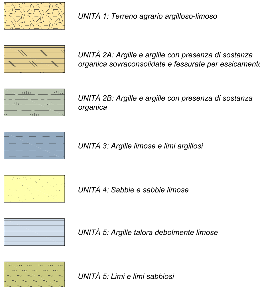
LEGENDA LITOLOGICA
