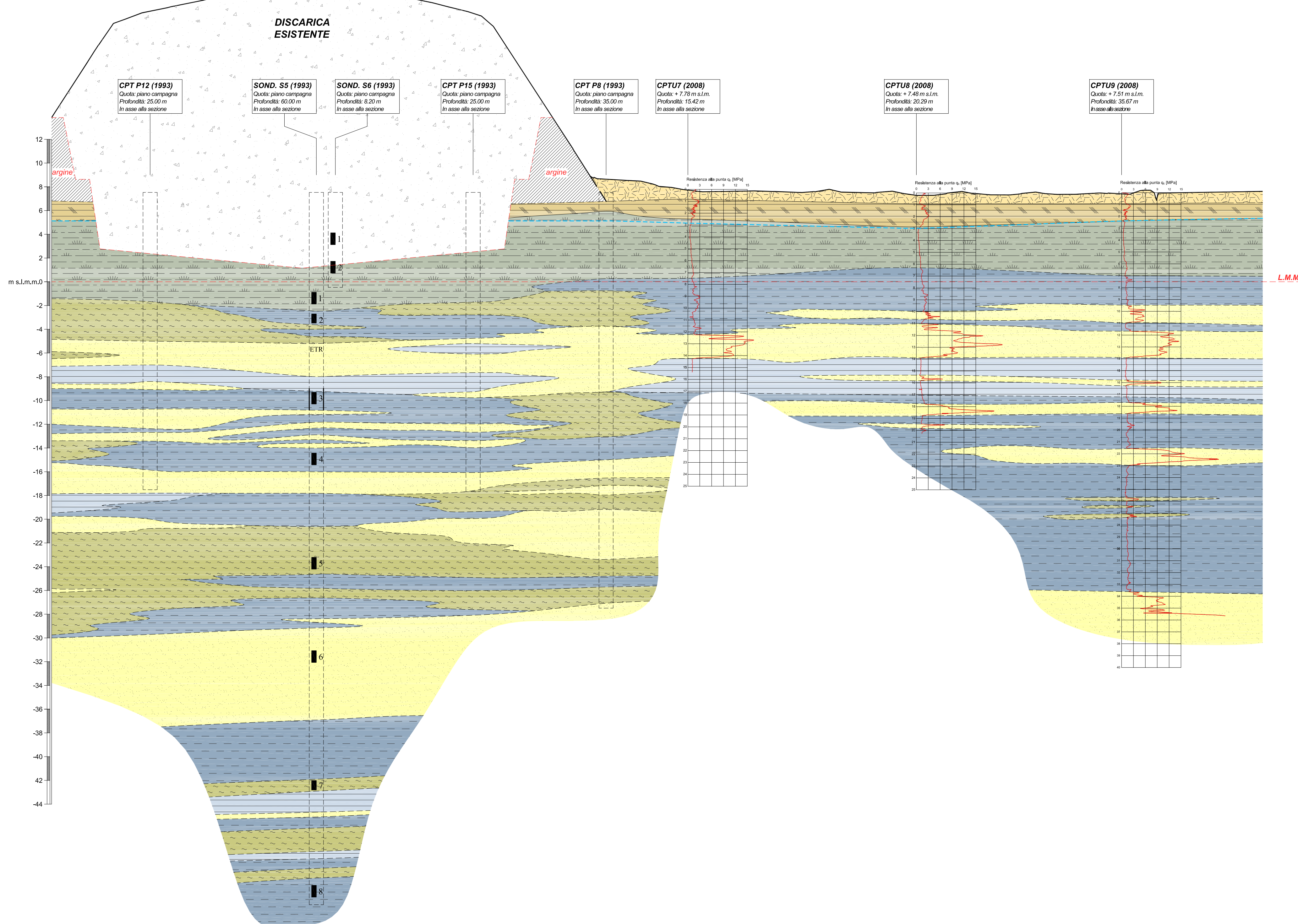
Sezione F-F' scala 1:1.000/200
