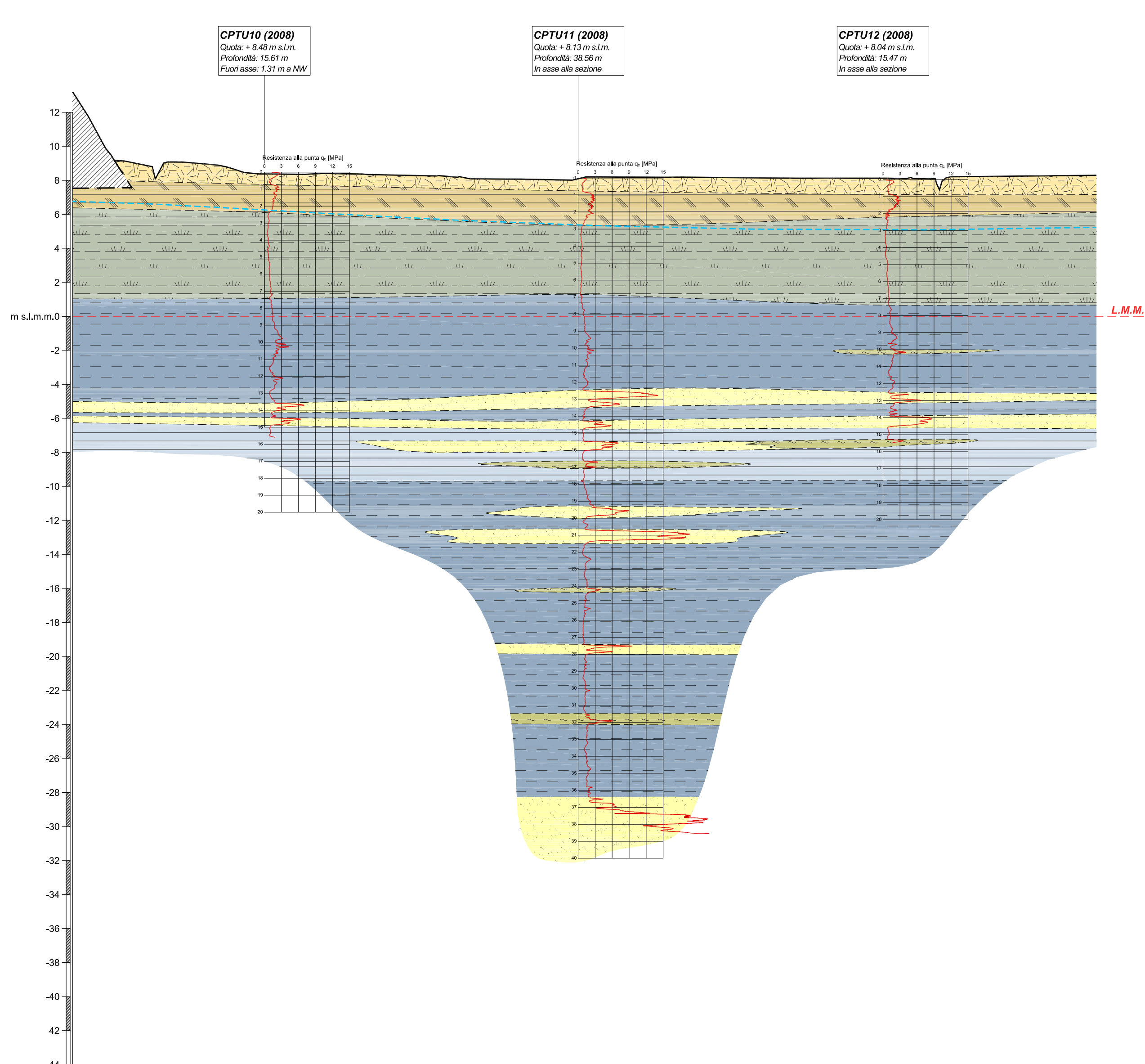
Sezione G-G' scala 1:1.000/200
