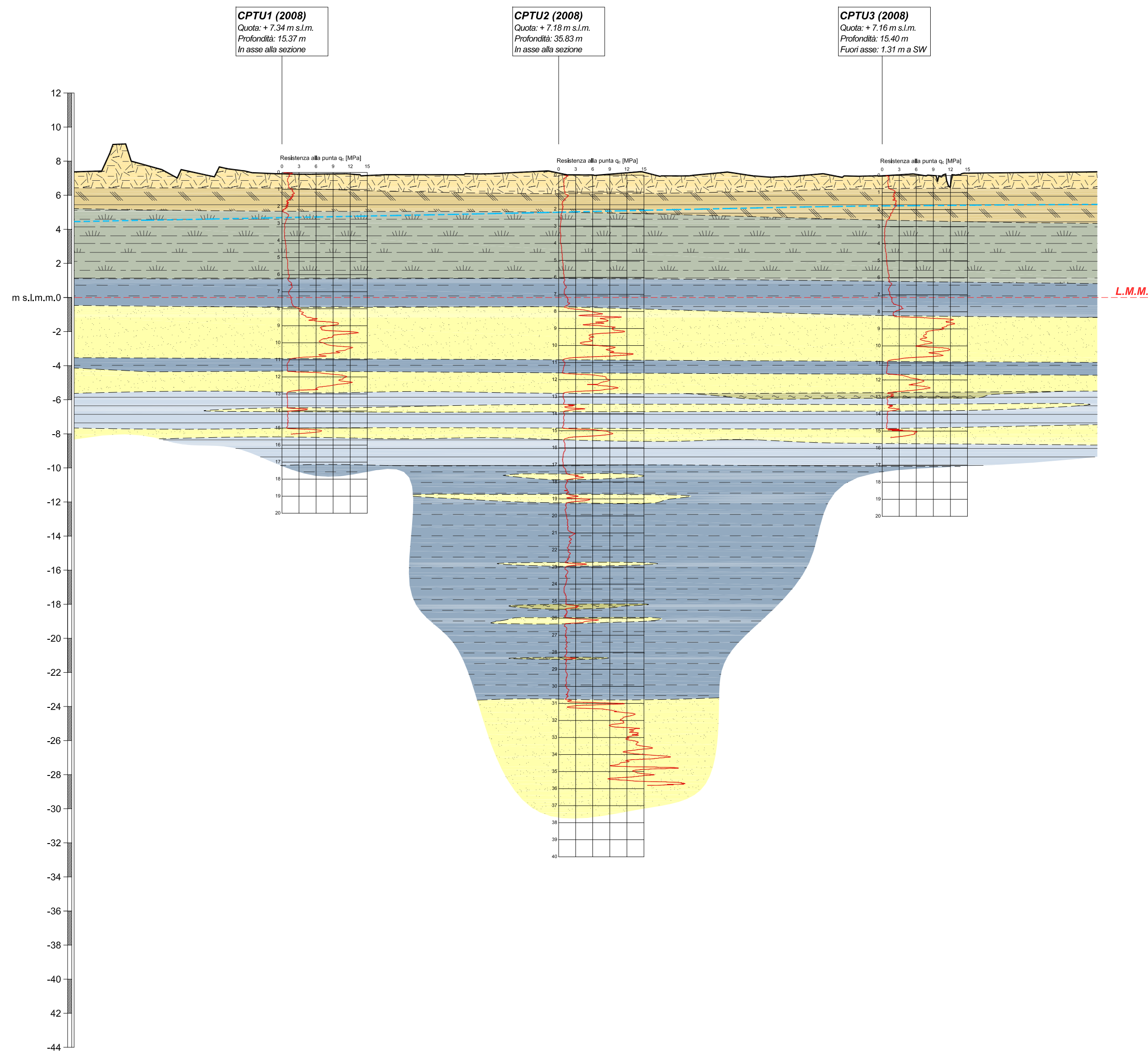
Sezione D-D' scala 1:1.000/200
