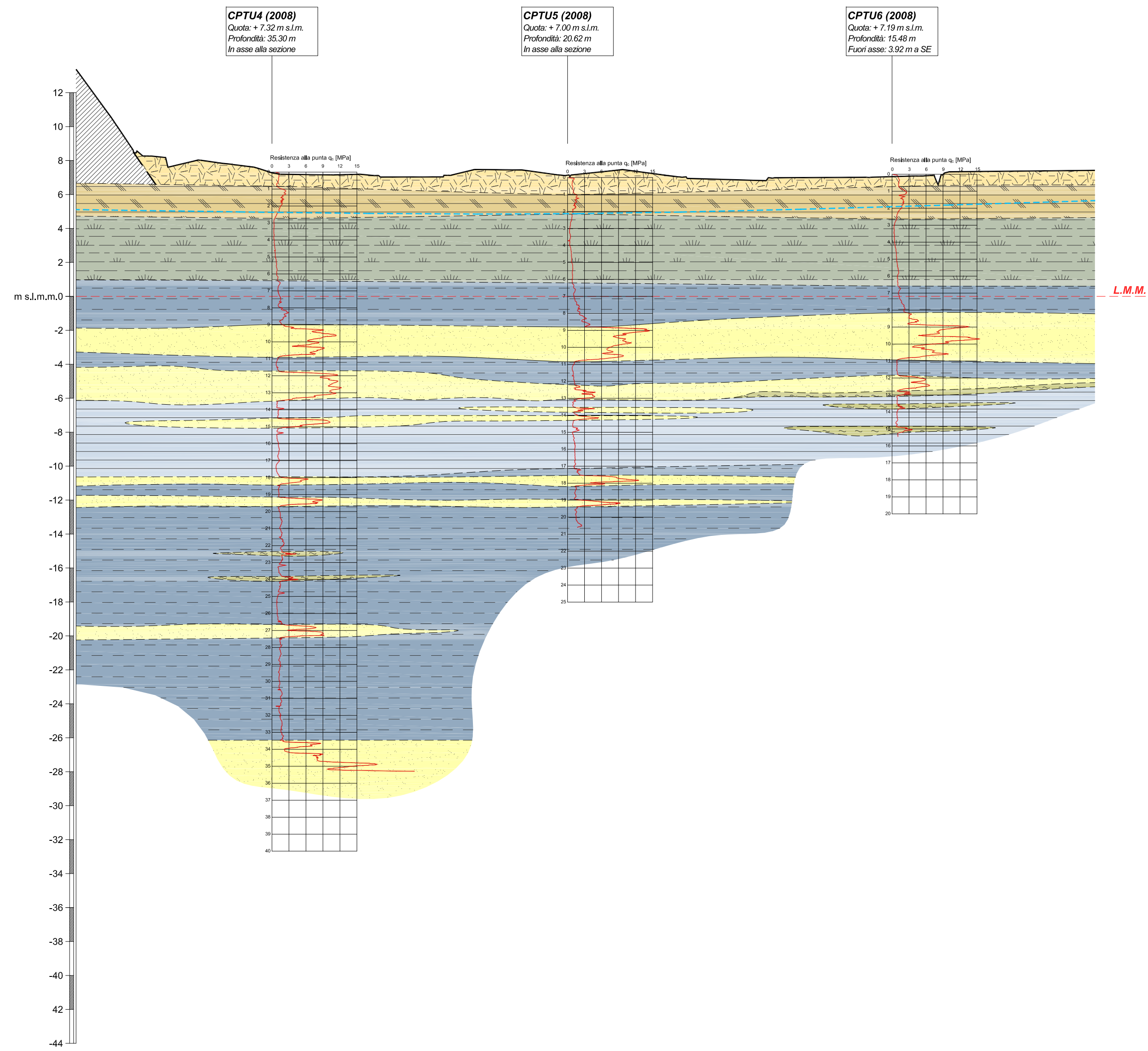
Sezione E-E' scala 1:1.000/200
