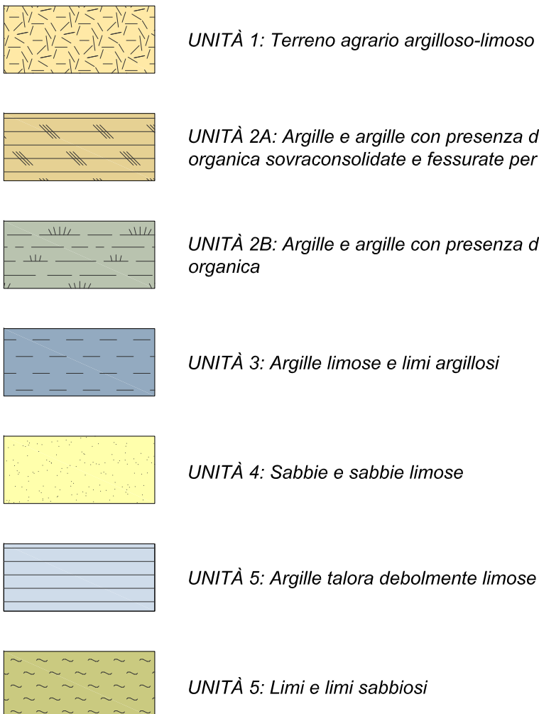
LEGENDA LITOLOGICA
