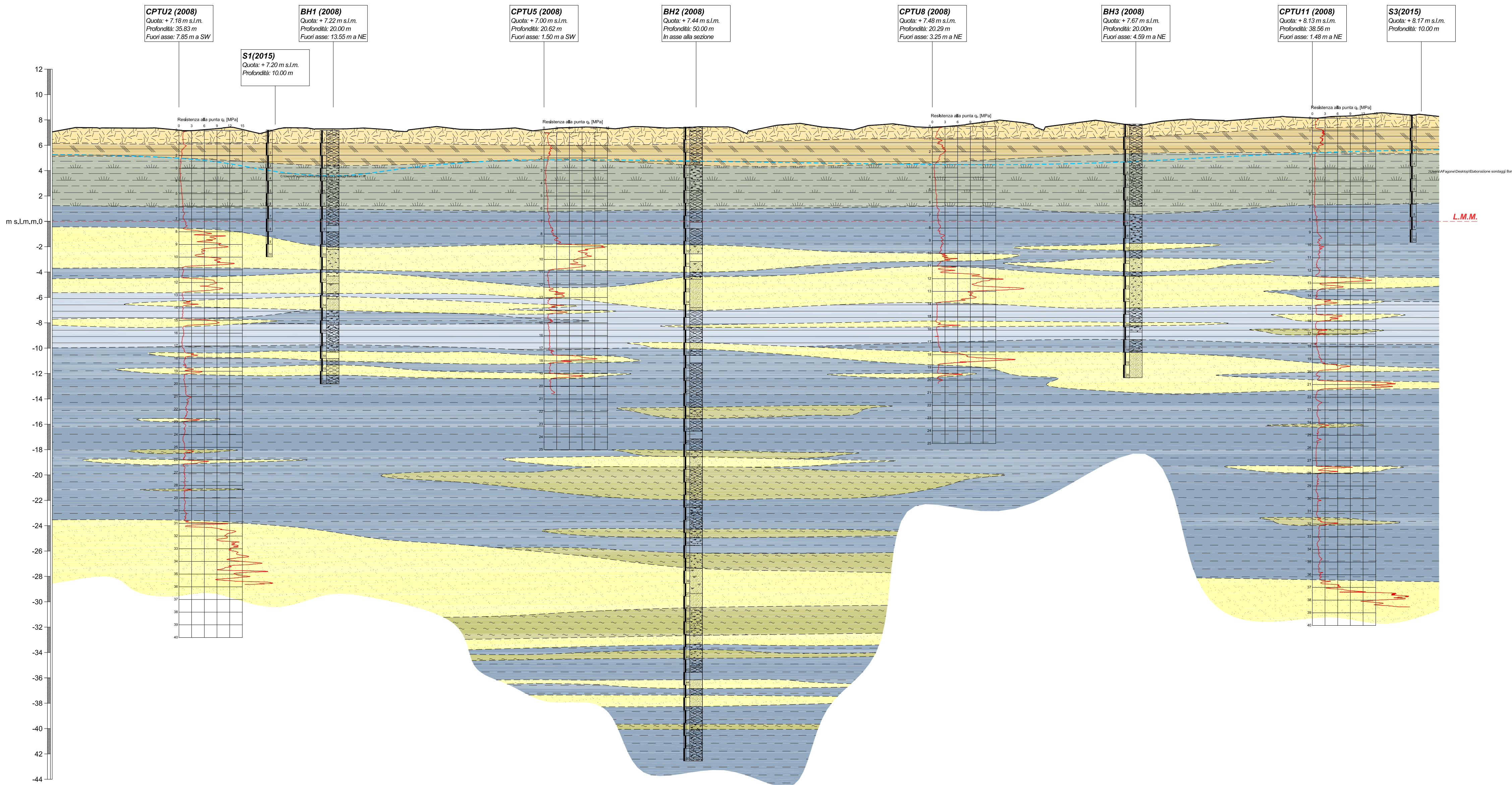
Sezione B-B' scala 1:1.000/200
